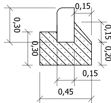
Detalē Nr. 2 M 1:20 Gatvės bordiūras
