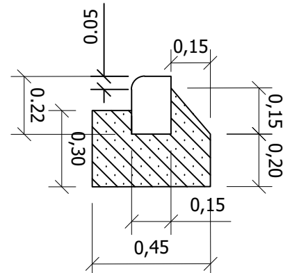
Detalē Nr. 3 M 1:20 Nužemintas gatvės bordiūras
